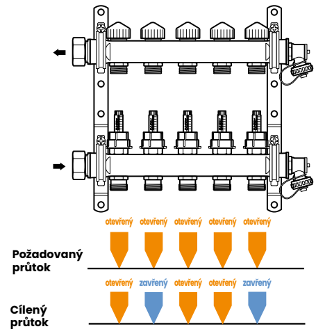
Uponor Vario S DFC rozdělovač sběrač
