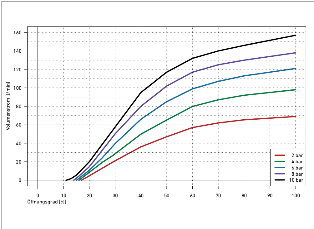
Spüleleistung DN15
