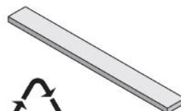
1005479 Uponor Tecto isolatiestrook EPS 11 mm Als warmte-isolatie met snijraster voor toepassing met uitvlakelementafdekfolie in het deur- en wandgebied.
