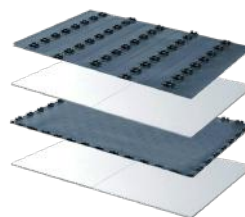
1016702 Uponor Nubos noppenplaat verdeler-/deurset EPS 11 Toepassen van de deurdoorvoer elementen in evenwijdige deuropeningen, door de eenvoudig op maat te snijden stroken. Per element zijn circa 10 stroken voor 5 deuropeningen te snijden.
