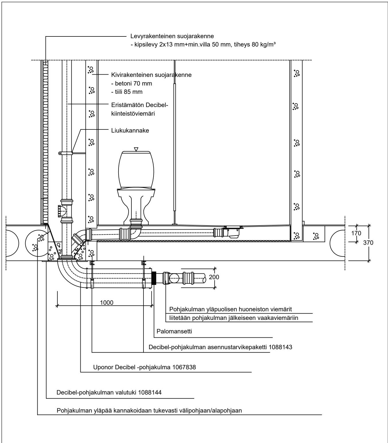
Kuva 22. Eristämättömän Uponor Decibel -kiinteistöviemärin äänitekniset suojarakenteet, äänitasovaatimus 28 dB(A). Pohjakulman yläpuolista huoneistoa palvelevia viemäriputkia ei liitetä pystykokoosviemäriin, vaan ne johdetaan alapohjan alapuolelle ja liitetään äänenvaimentimen jälkeiseen vaakaviemäriin.
