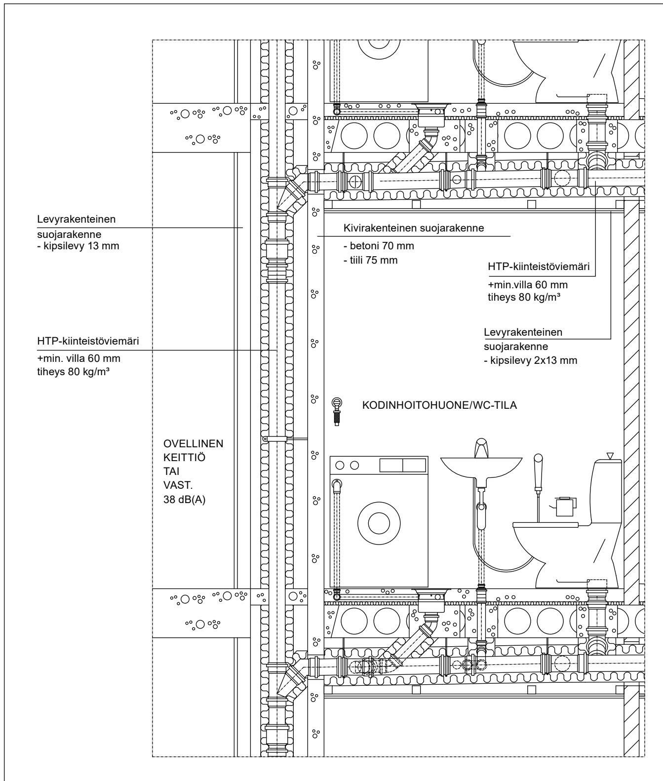
Kuva 13. Eristetyn Uponor HTP -kiinteistöviemärin äänitekniset suojarakenteet pohjakulman kahden yläpuolisen kerroksen yläpuolella (3. krs-), äänitasovaatimus 38 dB(A). El 30. Viemärijärjestelmien paloeristämisessä voidaan soveltaa esim. PAROC Hvac Fire -ilmakanavien paloeristysratkaisua, jolla saavutetaan palosuojaus ulkopuolista paloa vastaan. Paloeristysratkaisu tulee hyväksyttävä paikallisella rakennusvalvontaviranomaisella.
