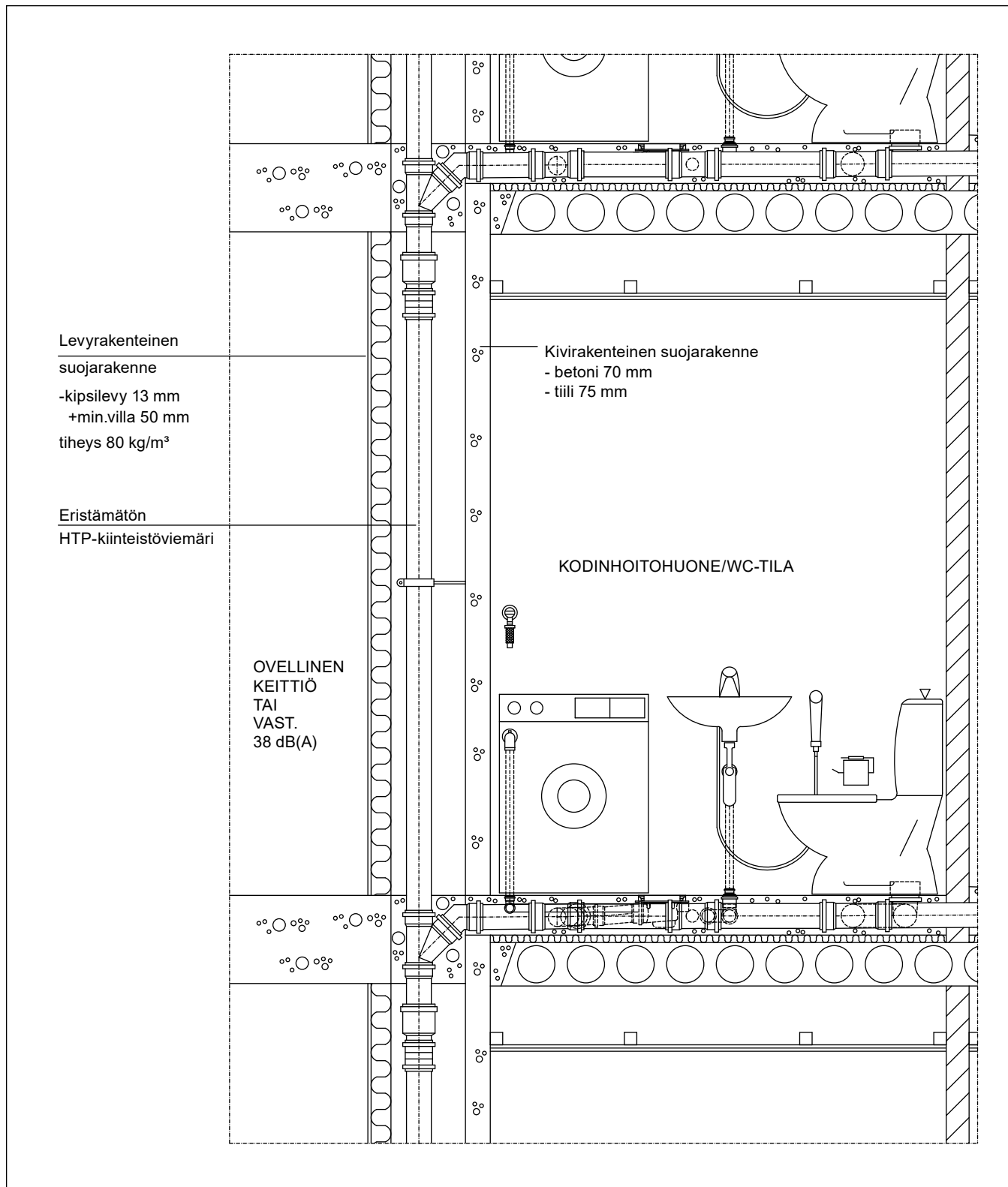
Kuva 11. Eistämättömän Uponor HTP -kiinteistöviemärin äänitekniset suojarakenteet pohjakulman kahden yläpuolisen (3. krs-) kerroksen yläpuolella, äänitasovaatimus 38 dB(A). EI 30.
