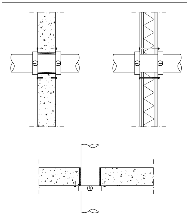
Kuva 82. Osastoivan rakenteen pintaan asennettava palomansetti seinä- ja lattiarakenteen läpivienneissä.
