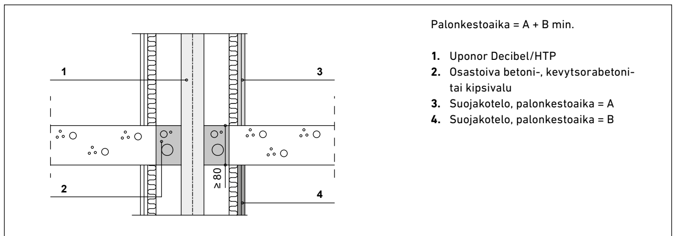
Kuva 23. Viemäriin läpiviennin kohdan ja suojarakenteen palonkestoajan määrittäminen.
