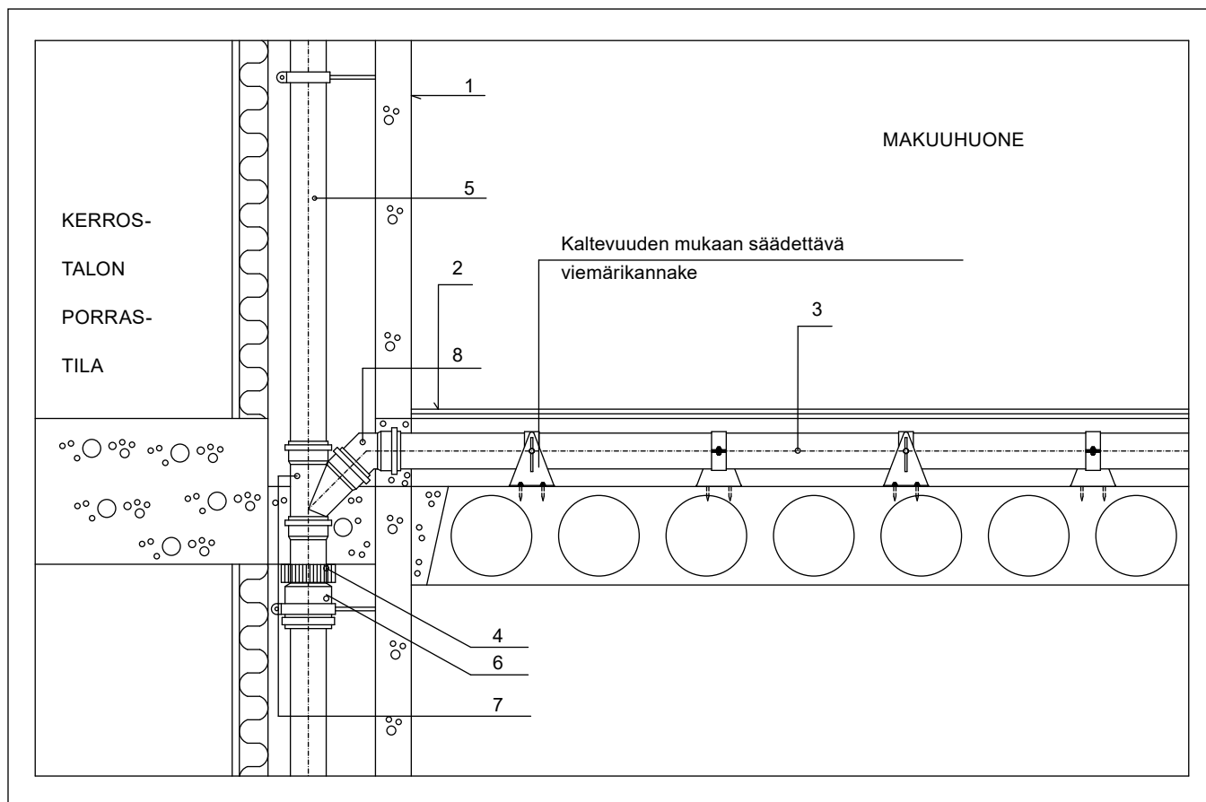
Kuva 21. Esimerkki kytkentä- ja vaakakokoojaviemärien asennuksesta ns. kerroslattian yhteydessä. Palomansetilla saavutetaan vaadittava palo-osastointiluokka.
