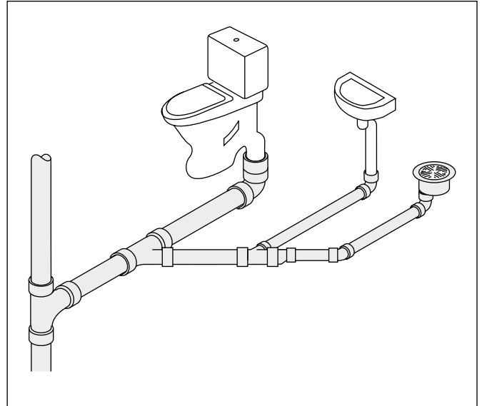
Kuva 65. Supistussyhteen asennus
