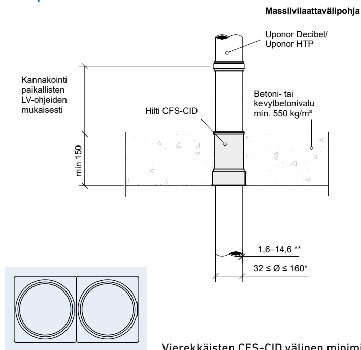
Kuva 28. Palo-osaston läpivienti massiivilaattaväliopohjassa – palokatkoite Hilti CFS-CID.
