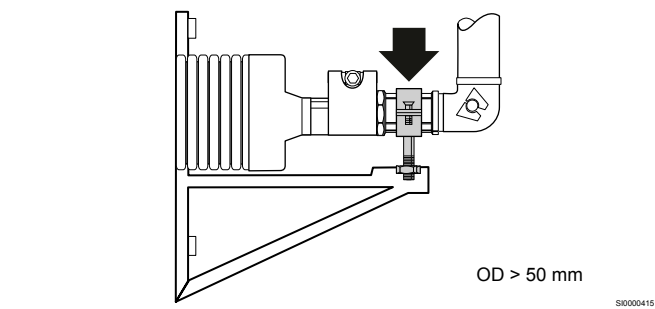
Анкеровка с помощью муфты места крепления Wipex (наружный диаметр > 50 мм)
