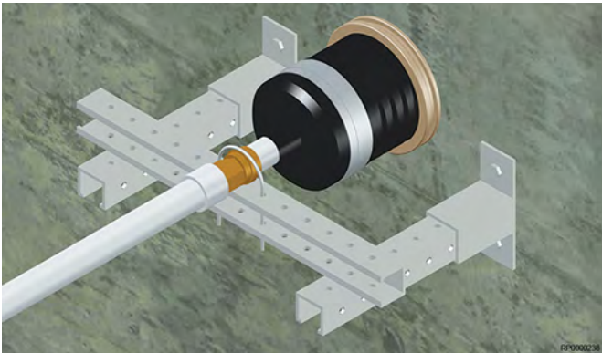
Анкеровка с помощью муфты места крепления Wipex (наружный диаметр > 50 мм)
