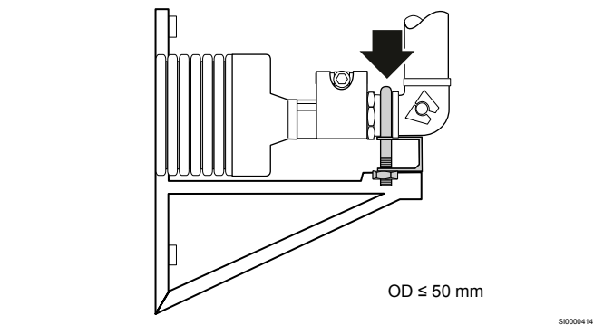
Анкеровка за фитинг (наружный диаметр ≤ 50 мм)
