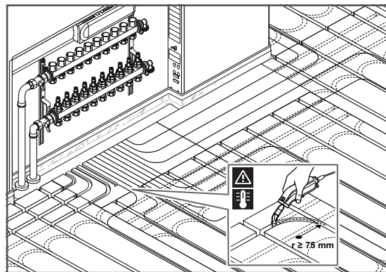
2. За необхідності виріжте додаткові пази.
