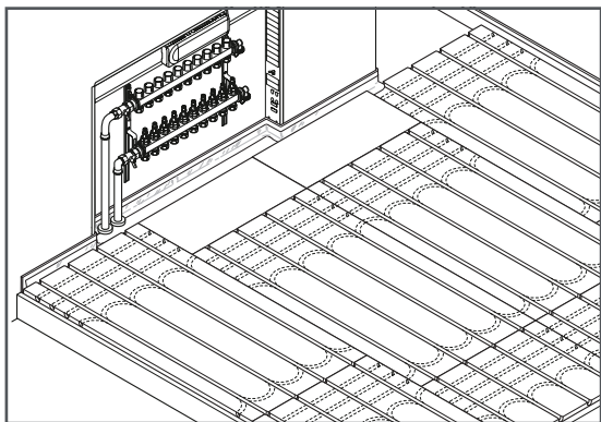
1. Укладіть панелі Siccus.
