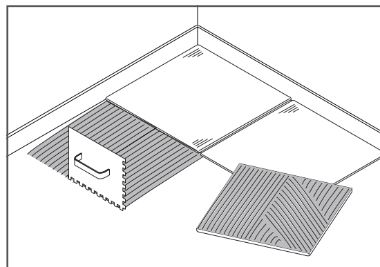
4. Безпосереднє укладання фінішного покриття на панелі відповідно до специфікації.
