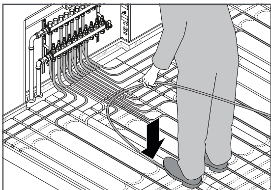
3. Прокладіть робочі труби Uponor.
