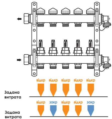
Колектор Uponor Vario S DFC
