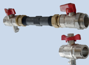
Горизонтальне підключення Vario HM 1'-1'; 1'-3/4'
