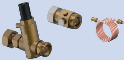
Регулятор тиску Vario
