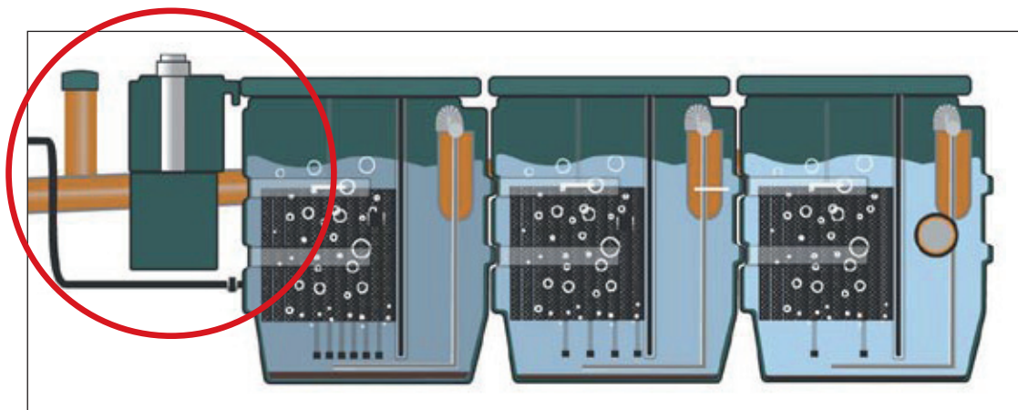
Teknikkassen sidder foran selve anlægget. I teknikkassen er alle de elektriske komponenter placeret.
