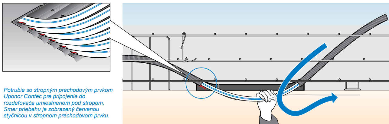
Uponor stropné prechodové prvky na debnení a tlakovú skúšku pripojovacích potrubí.
