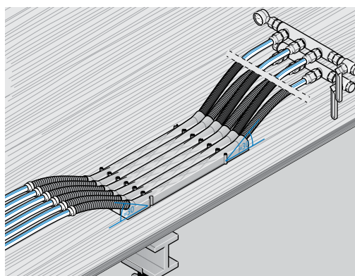
Uponor stropné prechodové prvky na debnení a tlakovú skúšku pripojovacích potrubí.
