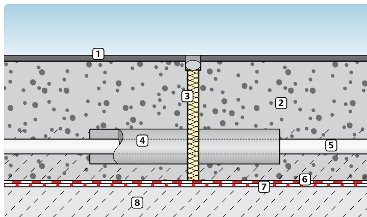
Schéma dilatácie škáry
