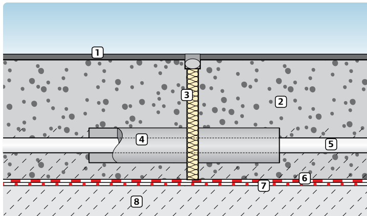
Schéma dilatáčnej škáry
