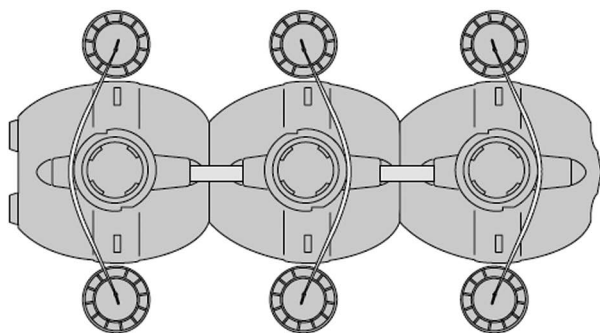
3m³ saostussäiliön ankkurointi
