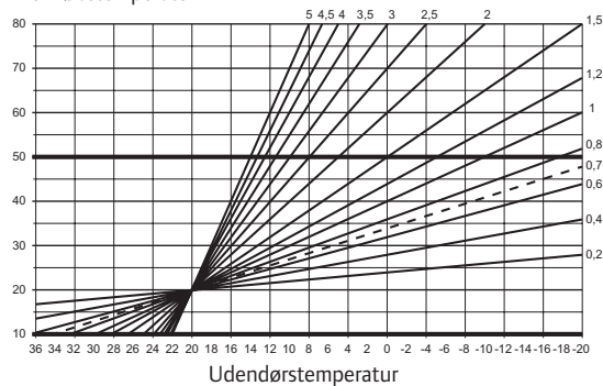
Fremløbstemperatur
