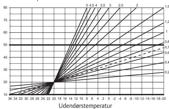
Fremløbstemperatur
