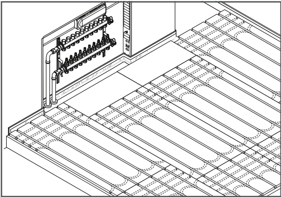
1. Išdėliojamos Siccus plokštės
