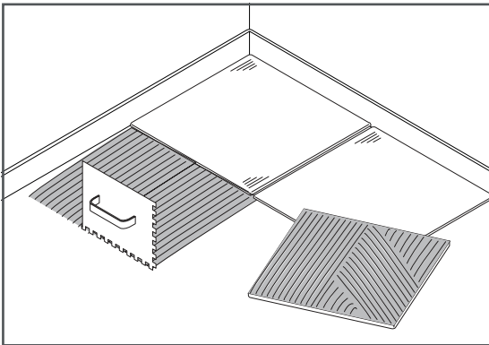
4. Klijuojamos plytelės (pagal gamintojo rekomendacijas)
