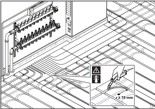
2. Išpjaunami trūkstami grioveliai
