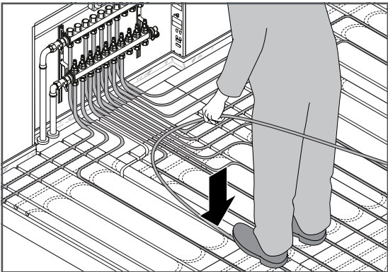
3. Išvedžiojami Uponor šildymo vamzdžiai
