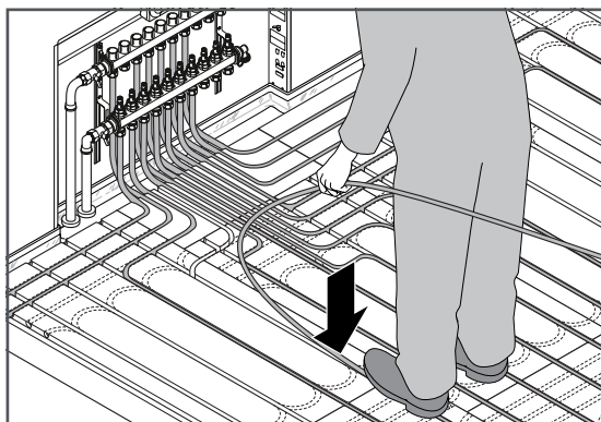
3. Namestitev ogrevalnih cevi Uponor
