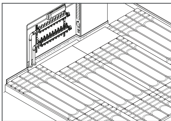
1. Vgradnja plošč Siccus
