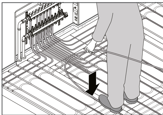
3. Nainstalujte topné potrubí Uponor
