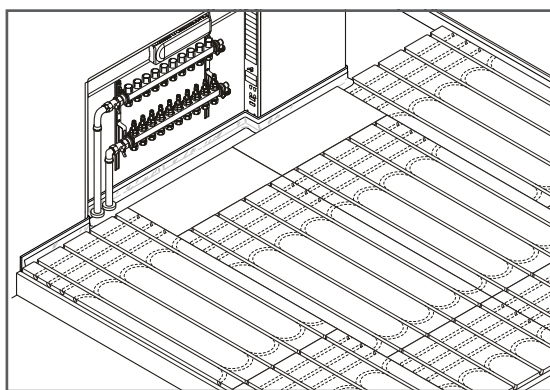
1. Nainstalujte panely Siccus
