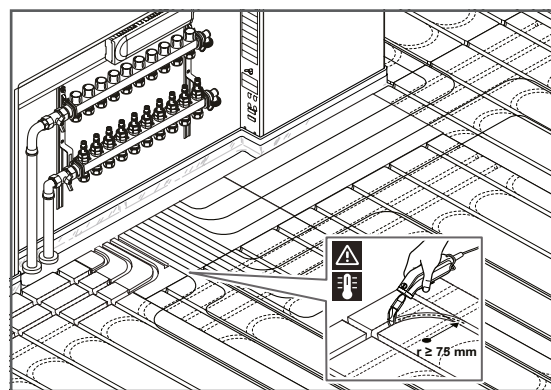
2. Vyřízněte chybějící drážky
