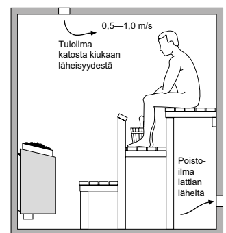
Löylyhuoneen ilmanvaihto
